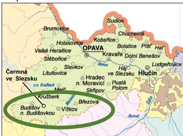
Mapa lokalizace obcí 3
